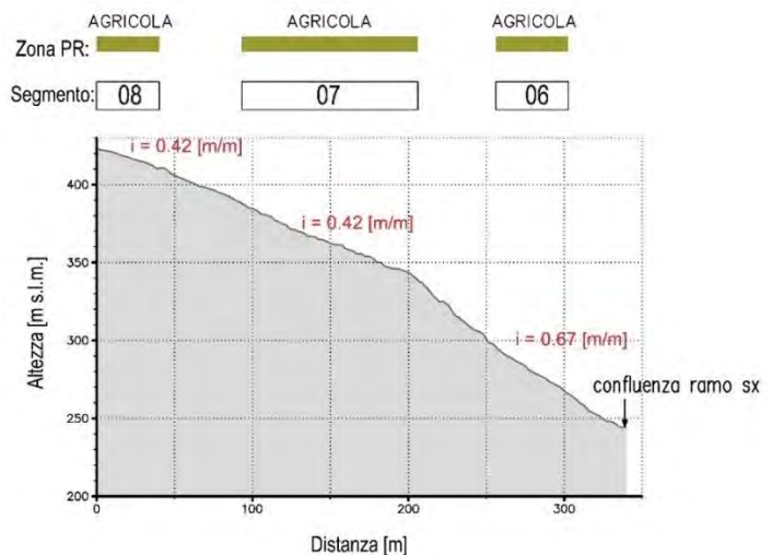
Fig. 17 Profilo longitudinale del riale Vignora (ramo sinistro e tratto di valle) con indicazione delle pendenze, dei tratti del rilievo ecomorfologico e delle zone agricole.
