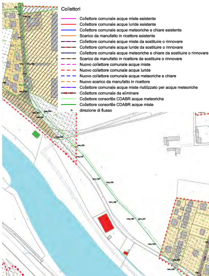
Fig. 10 Estratto della planimetria di riferimento del PGS di Bellinzona per il tratto SALEGGI_05 e foto dell'uscita del tubo in corrispondenza del gattile di Prato Carasso (parcella 393 RFD di Bellinzona).
