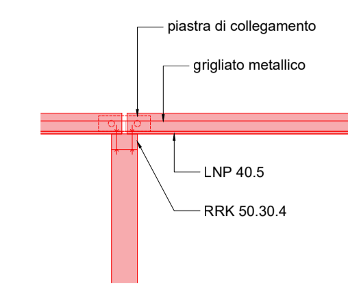
Dettaglio A - 1:20
