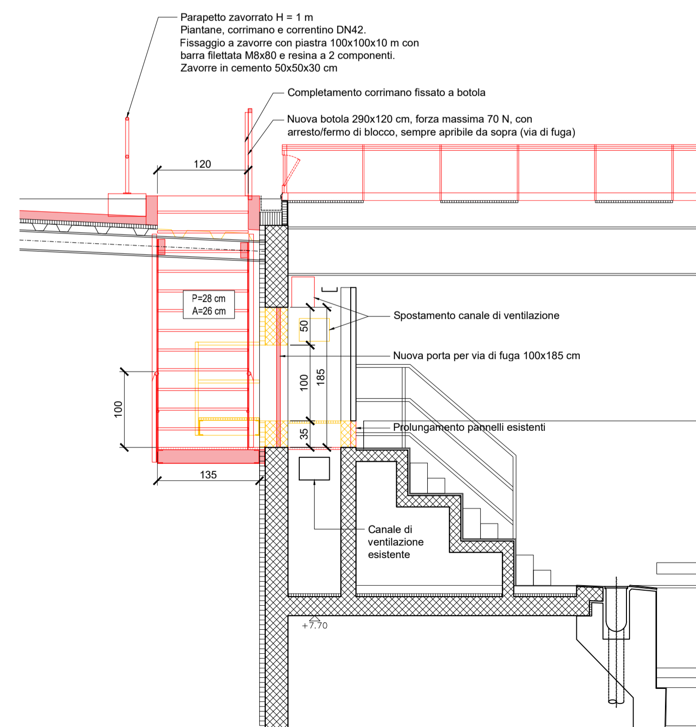
Sezione accesso tetto da piscina - 1:50
