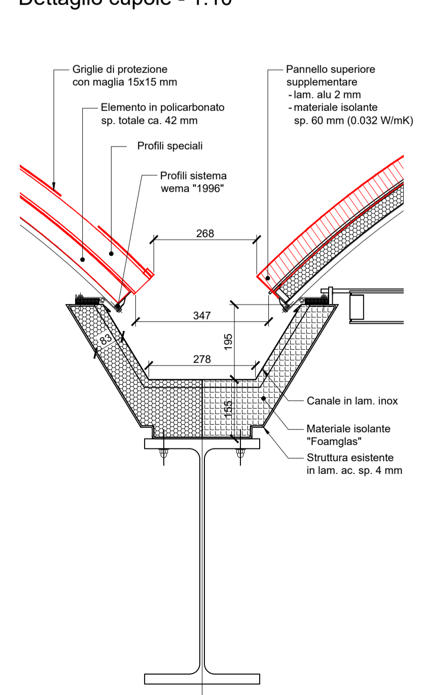
Dettaglio cupole - 1:10
