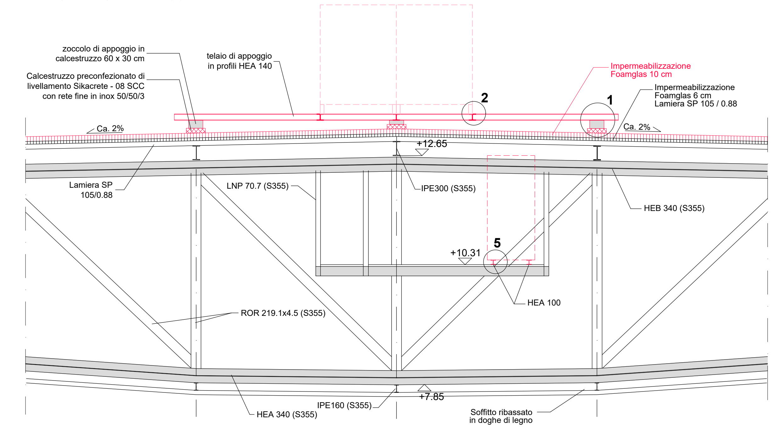
SEZIONE TRASVERSALE 1:50
