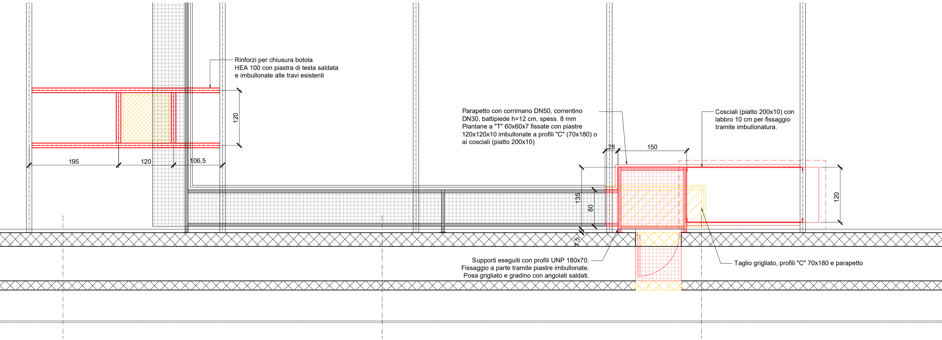
Pianta rinforzi botola esistente e nuova scala a tetto - 1:50
