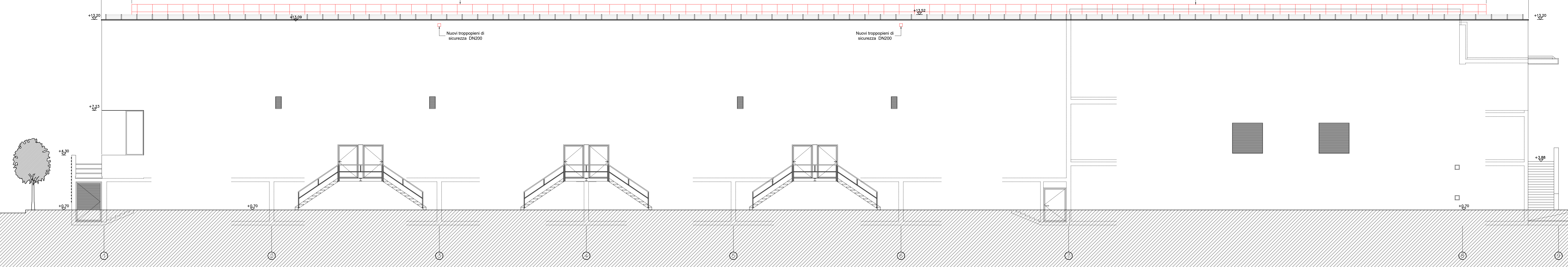
Dettaglio cupole - 1:20
