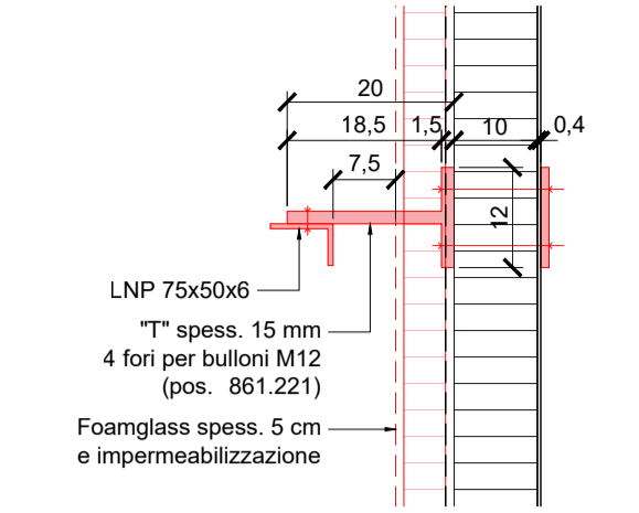
Dettaglio B - 1:20
