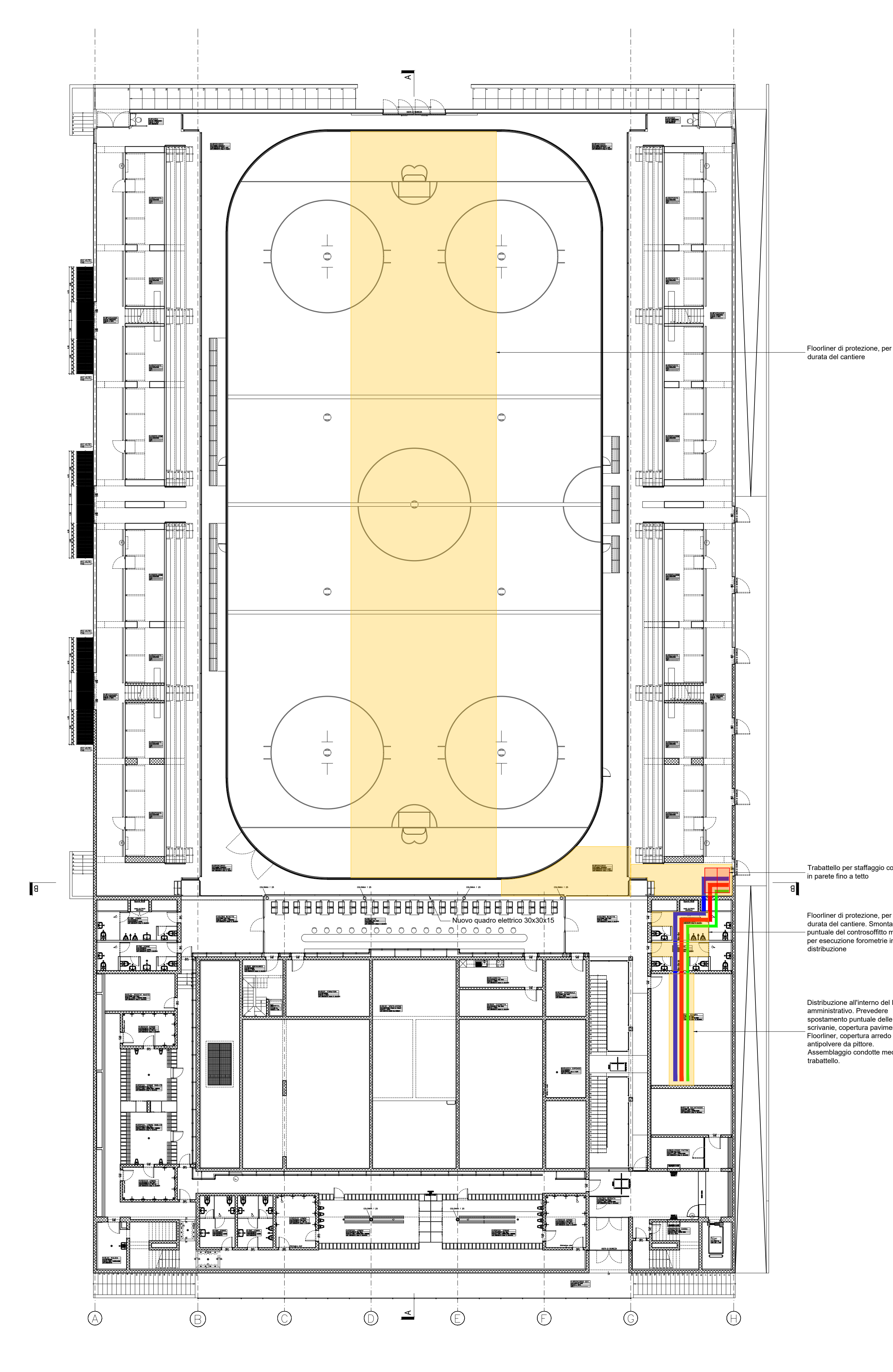
P1 - 1:200
