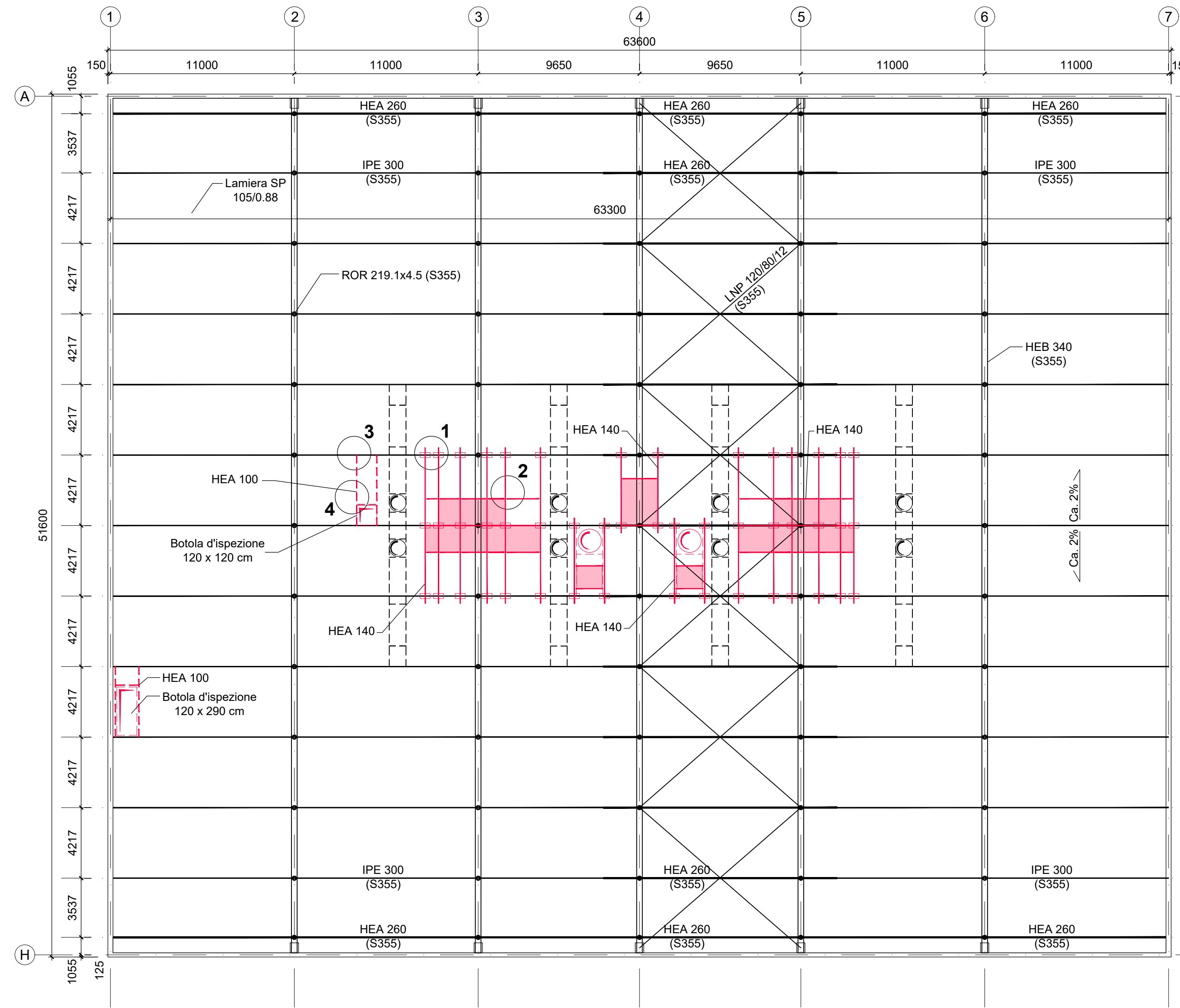
PIANTA INTERVENTO TETTO 1:100
