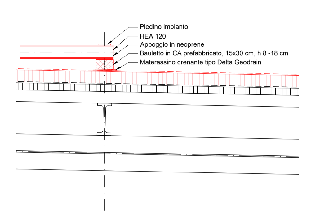
Dettaglio B - Travi d'appoggio impianti - 1:20
