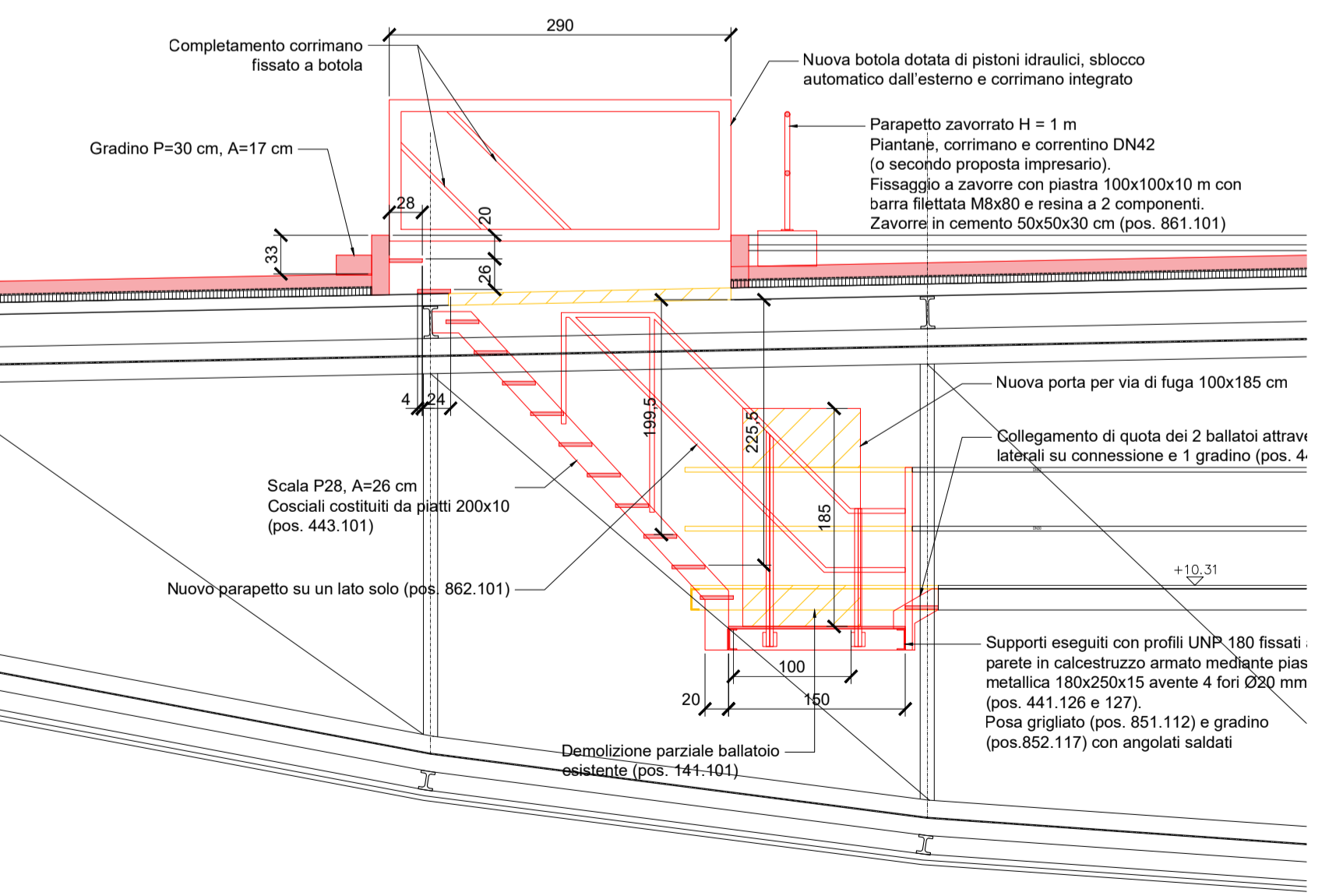
Sezione accesso tetto da piscina - 1:50
