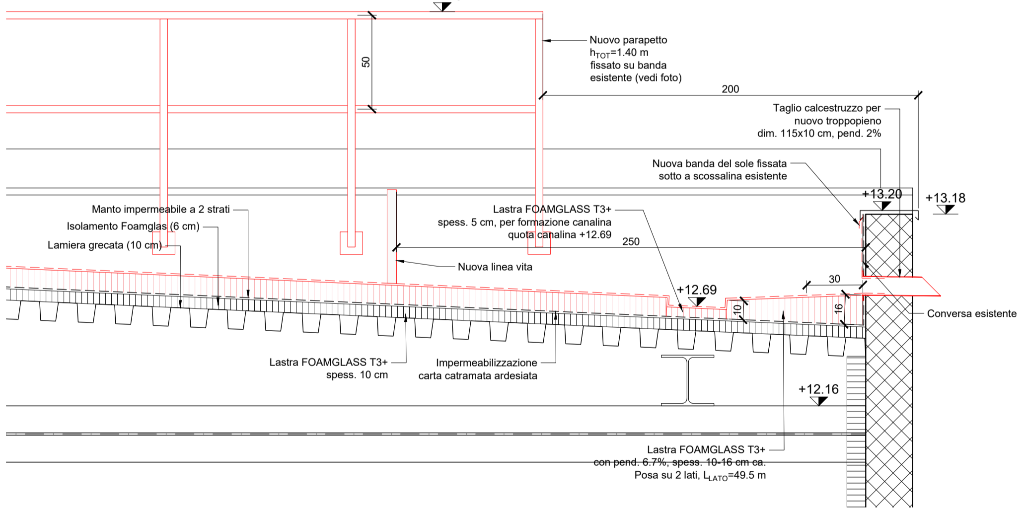
Dettaglio E - Nuovo troppopieno e parapetto - 1:20
