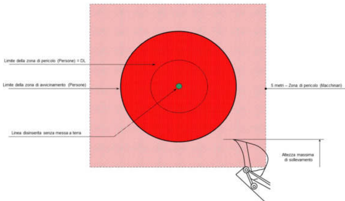
Figura 17: Lavori di costruzione/forestali in prossimità di linee elettriche disinserte e all'interno della zona di pericolo di 5 metri senza messa a terra per lavori e sotto supervisione continua
