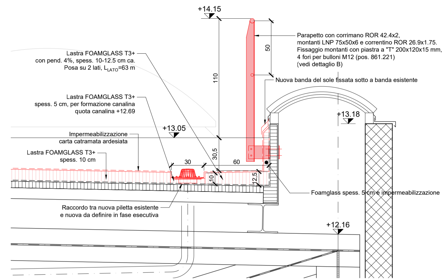
Sezione camminamento su cupole - 1:20
