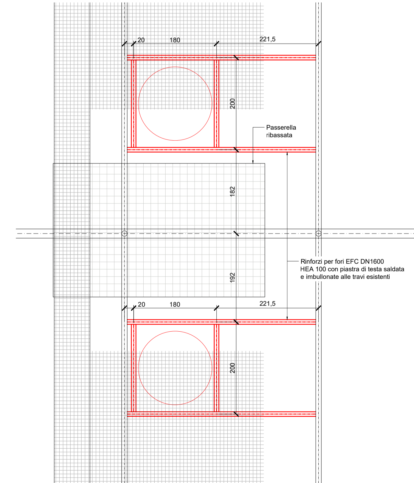
Pianta rinforzi fori EFC - 1:50
