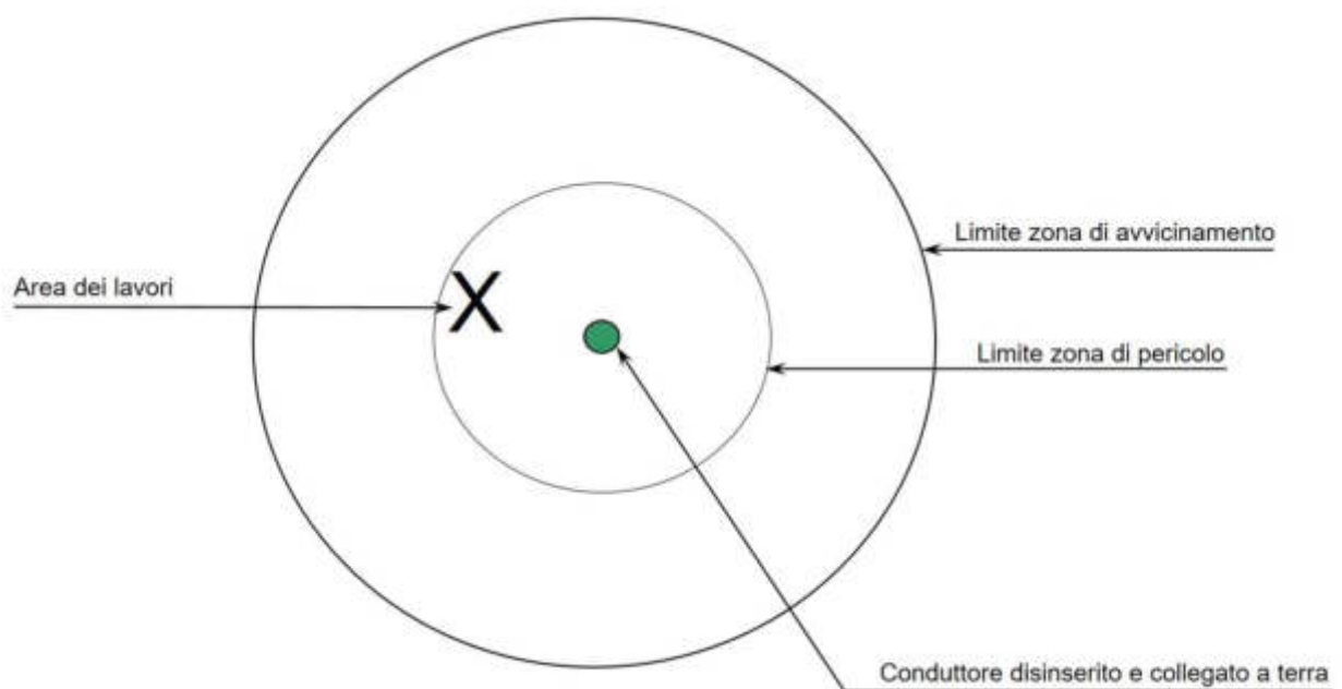
Figura 8: Lavori su linea elettrica disinserita
