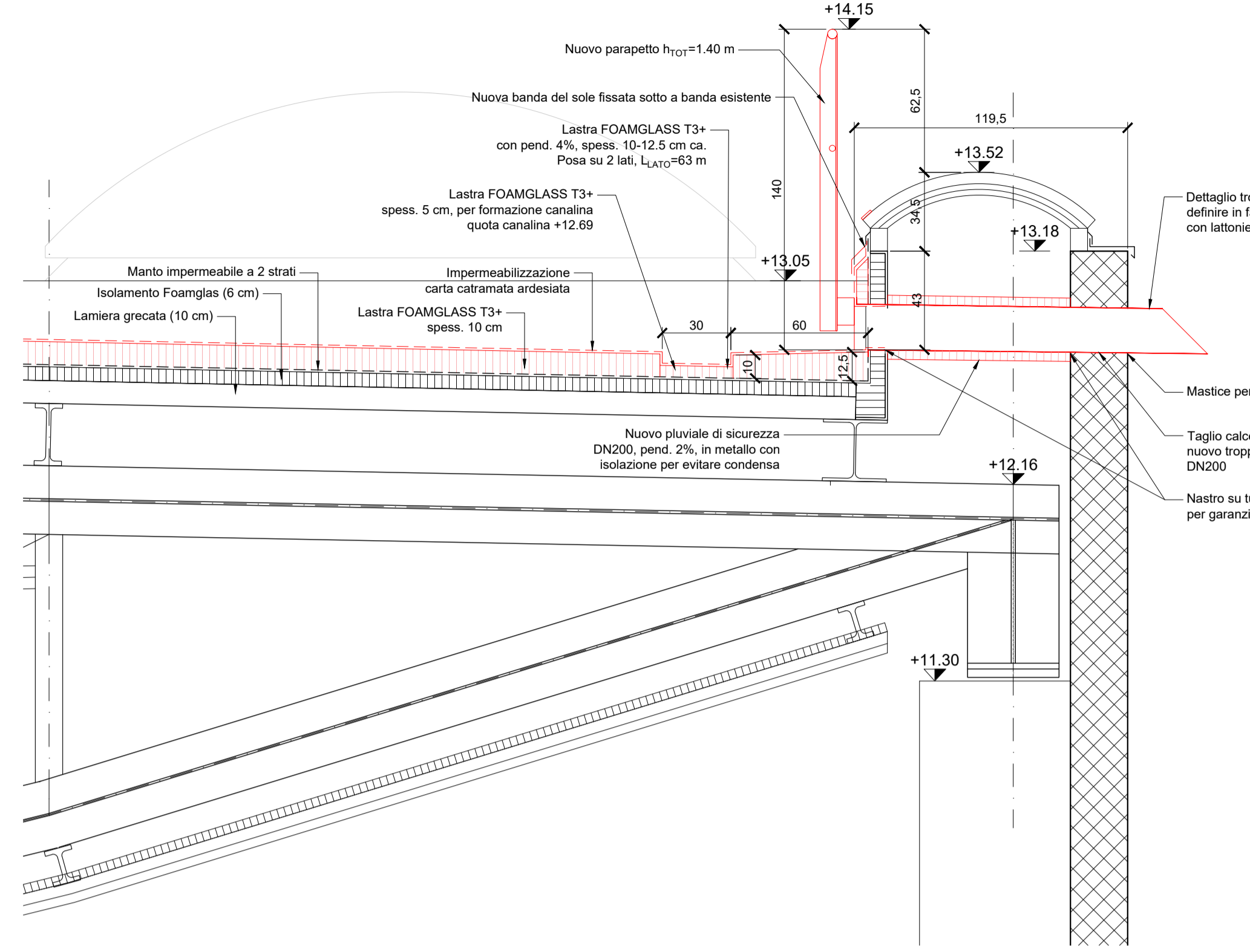
Dettaglio A - Nuovo troppopieno di sicurezza - 1:20
