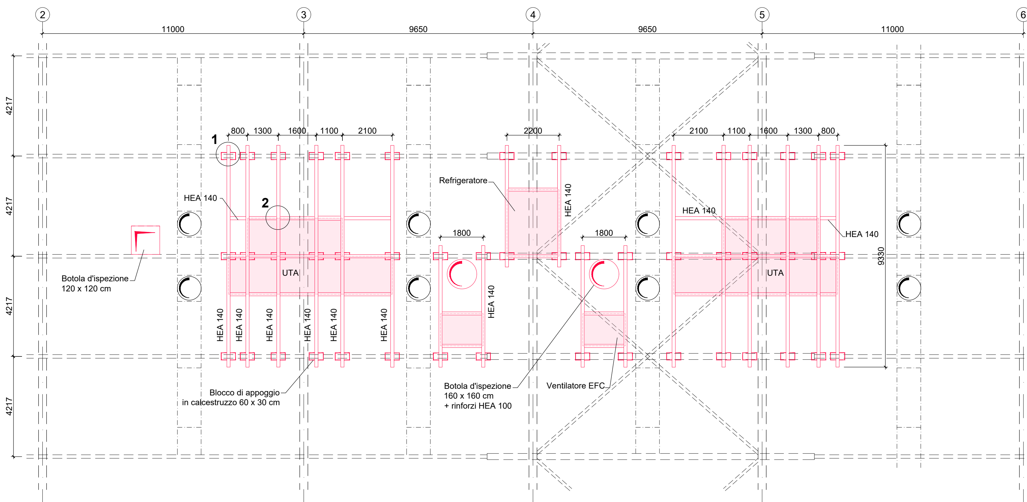
PIANTA INTERVENTO TETTO 1:100
