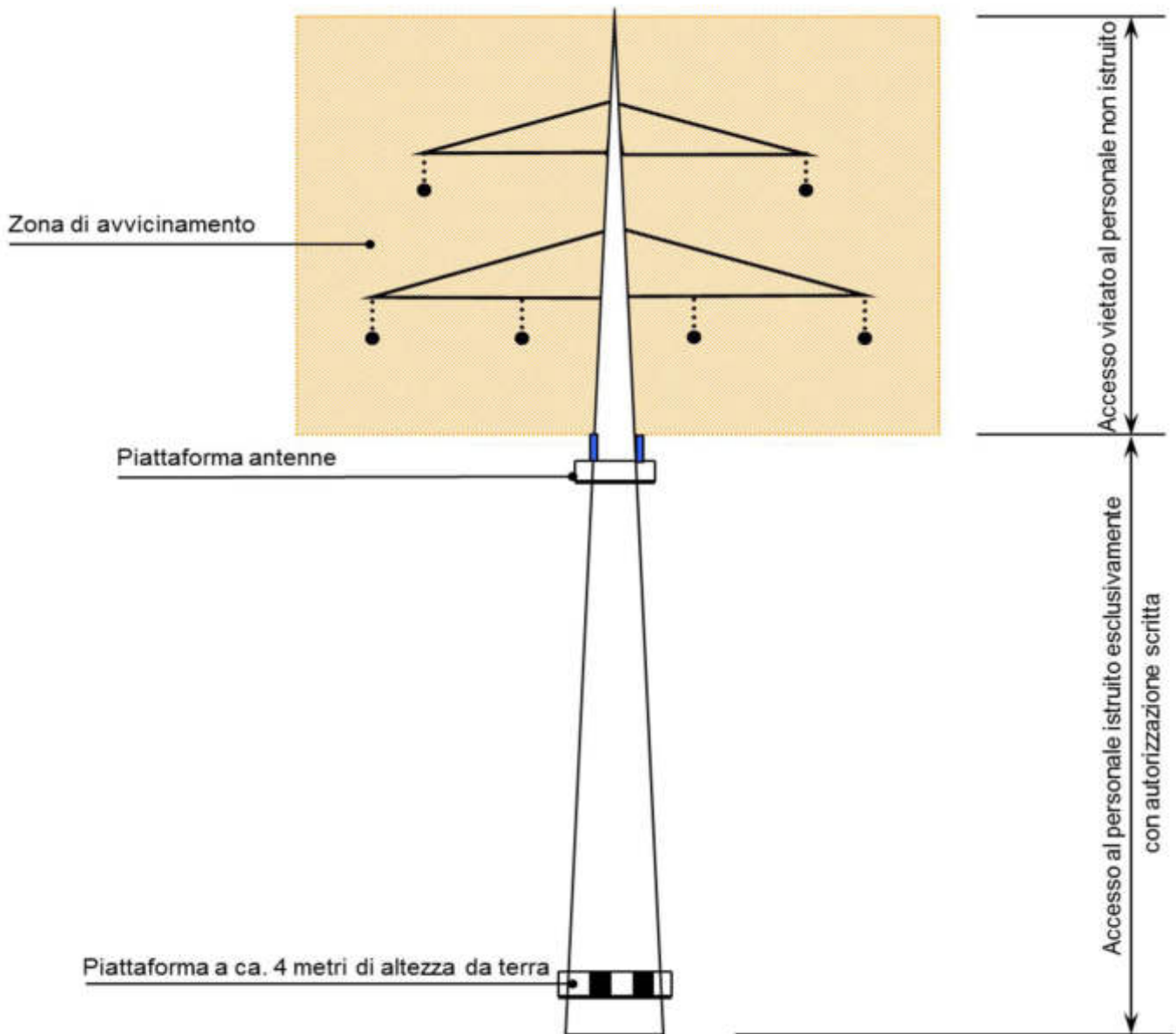
Figura 19: Schema di traliccio dell'alta tensione con sede di montaggio dell'antenna
