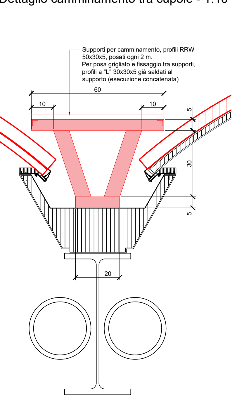
Dettaglio camminamento tra cupole - 1:10
