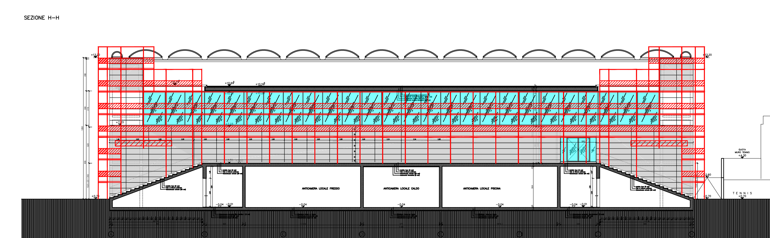
P1 - 1:200
