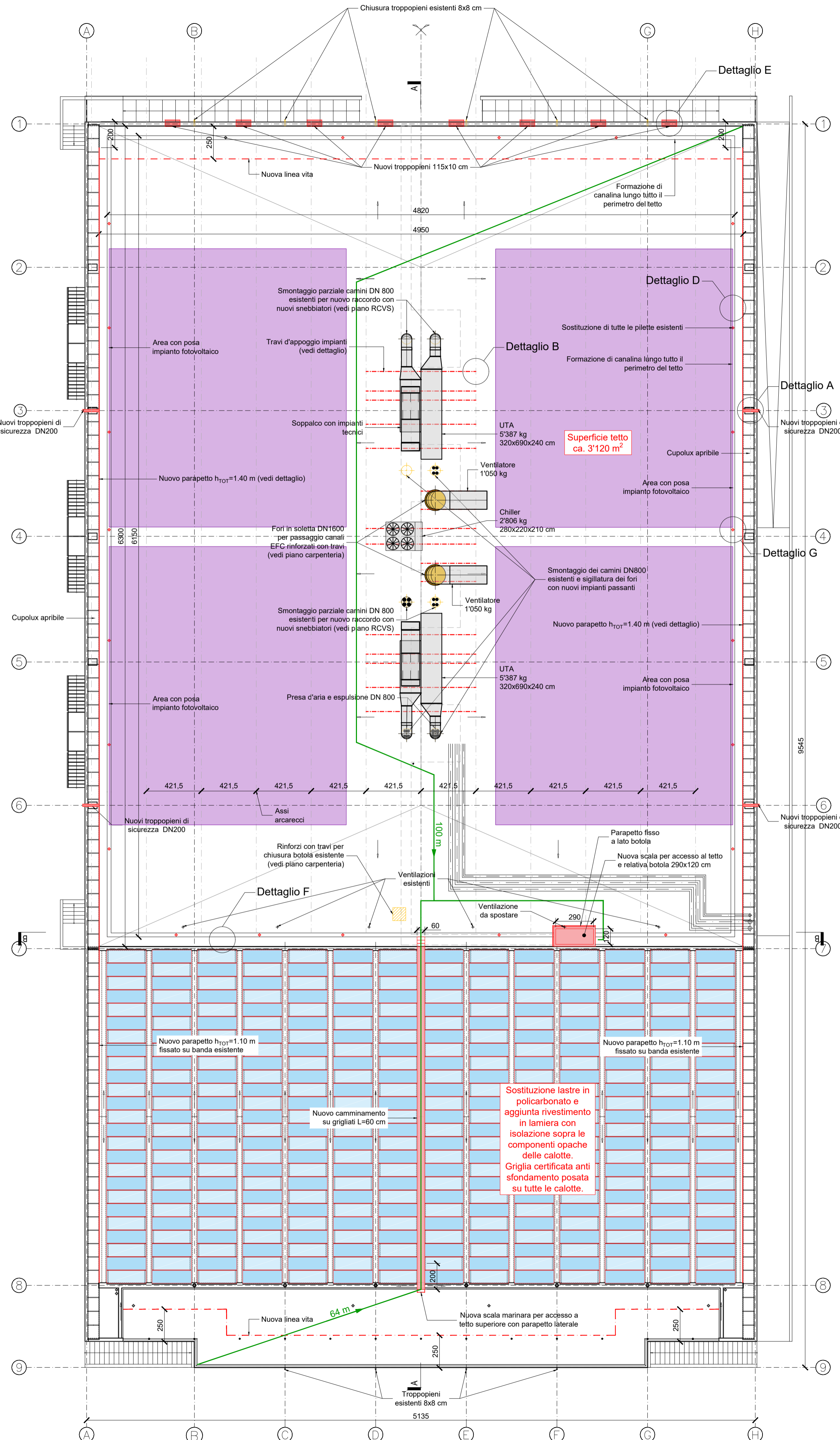
Pianta tetto - 1:200
