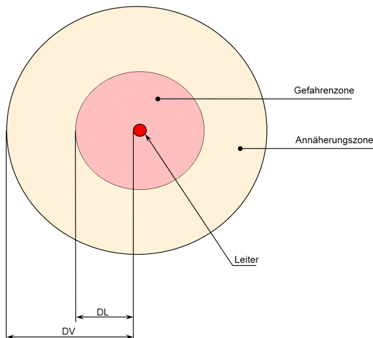
Figura 6: Schema delle distanze e zone per le persone, in riferimento alle LT e alla LC
