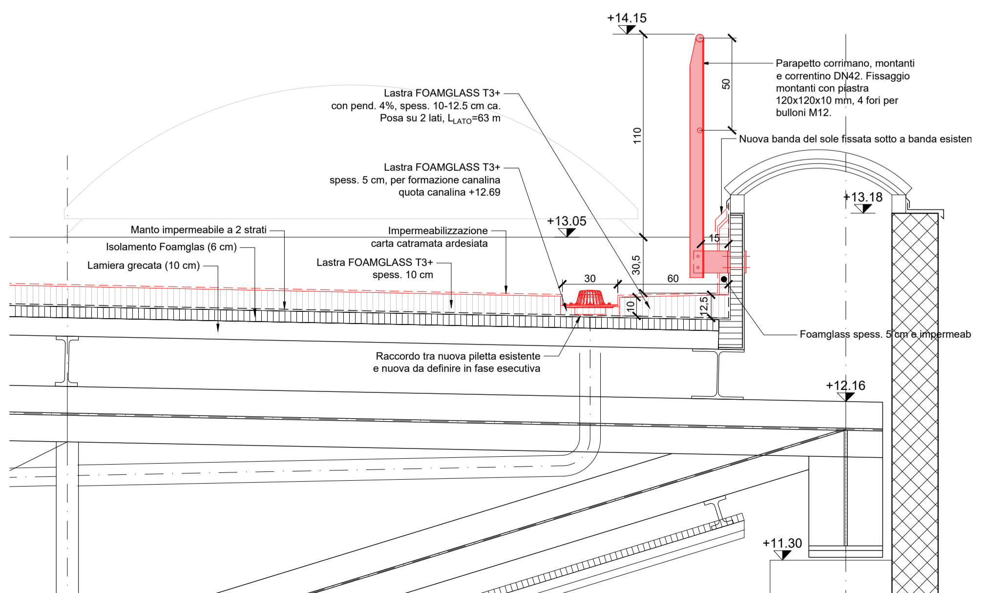
Dettaglio G - Nuova piletta - 1:20
