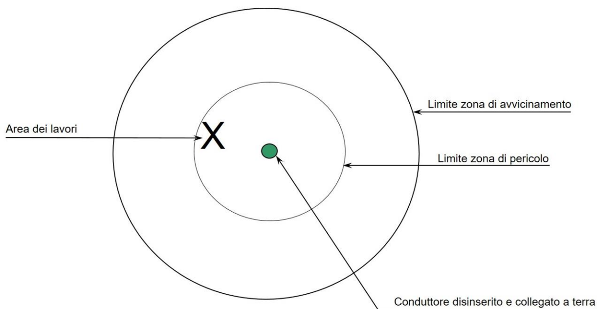
Figura 8: Lavori su linea elettrica disinserita
