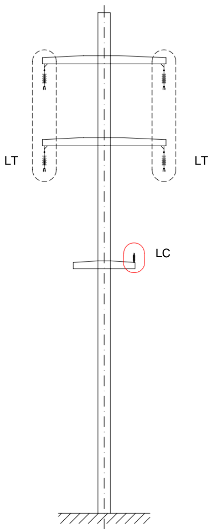
Figura 4: Linee elettriche sul tracciato dell'impianto di distribuzione della corrente di trazione (caso 1)
