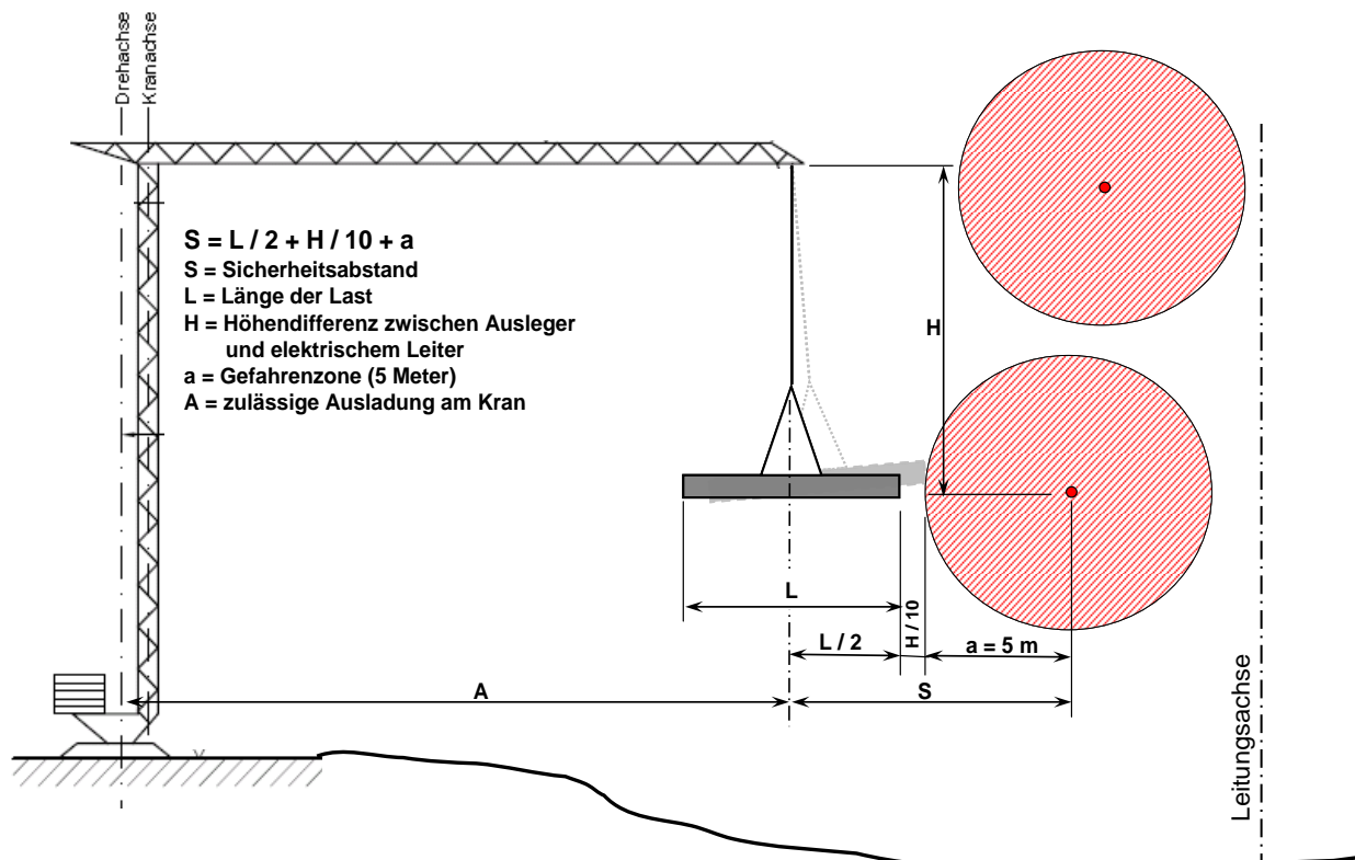
Figura 7: Esempio di rispetto della distanza di sicurezza con gru installata in prossimità di linee aeree FFS
