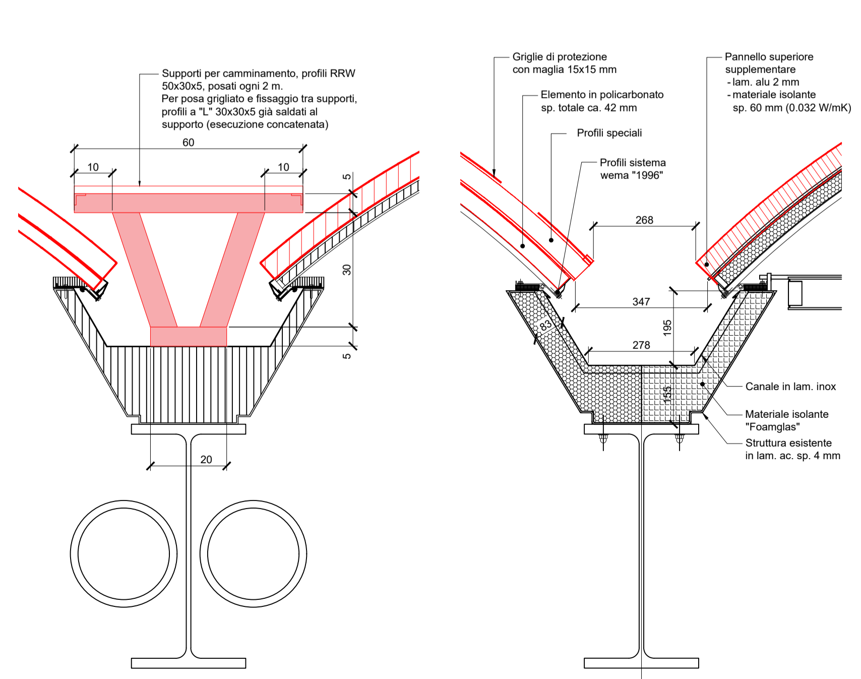
Dettaglio camminamento tra cupole - 1:10
