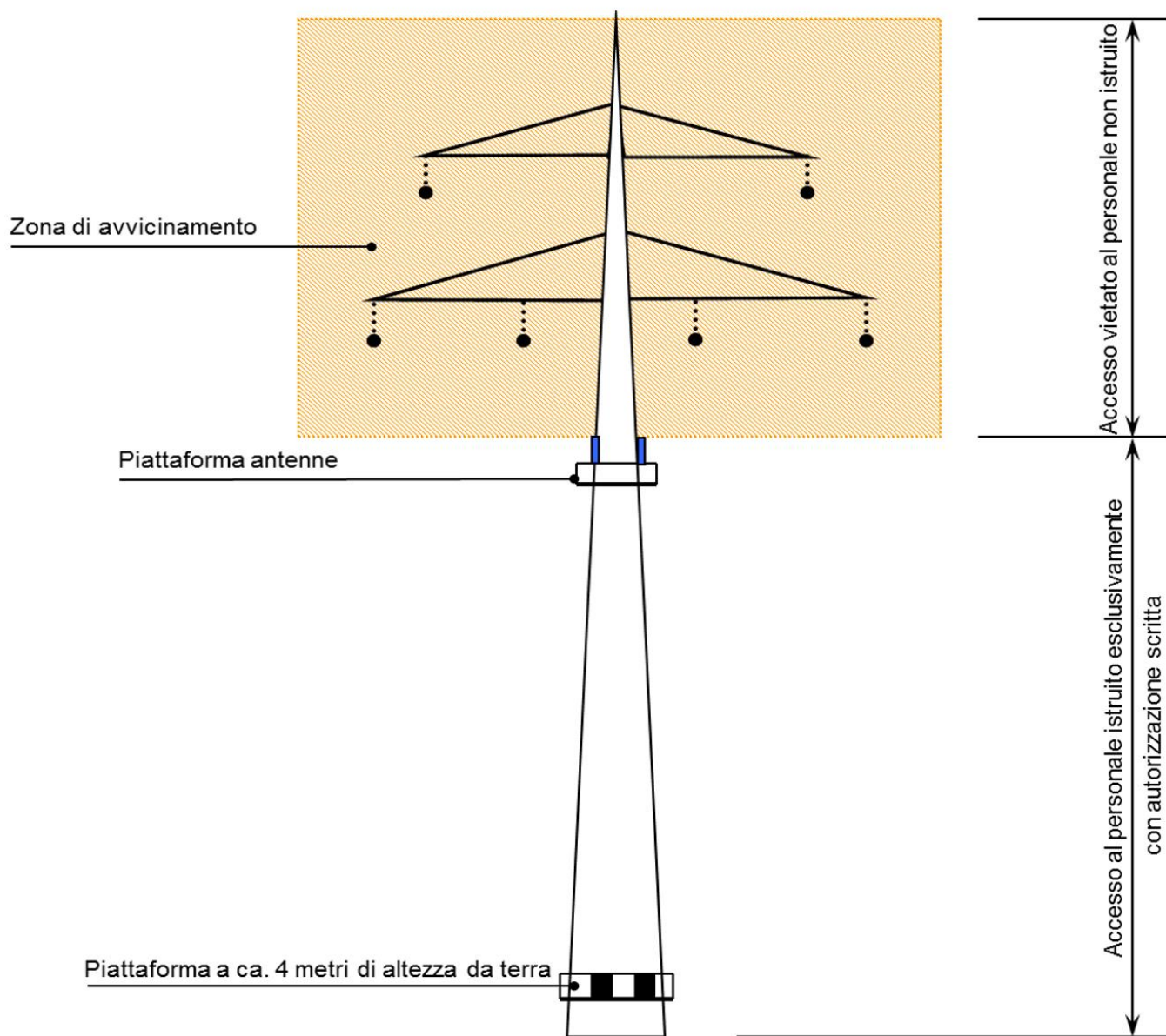
Figura 19: Schema di traliccio dell'alta tensione con sede di montaggio dell'antenna
