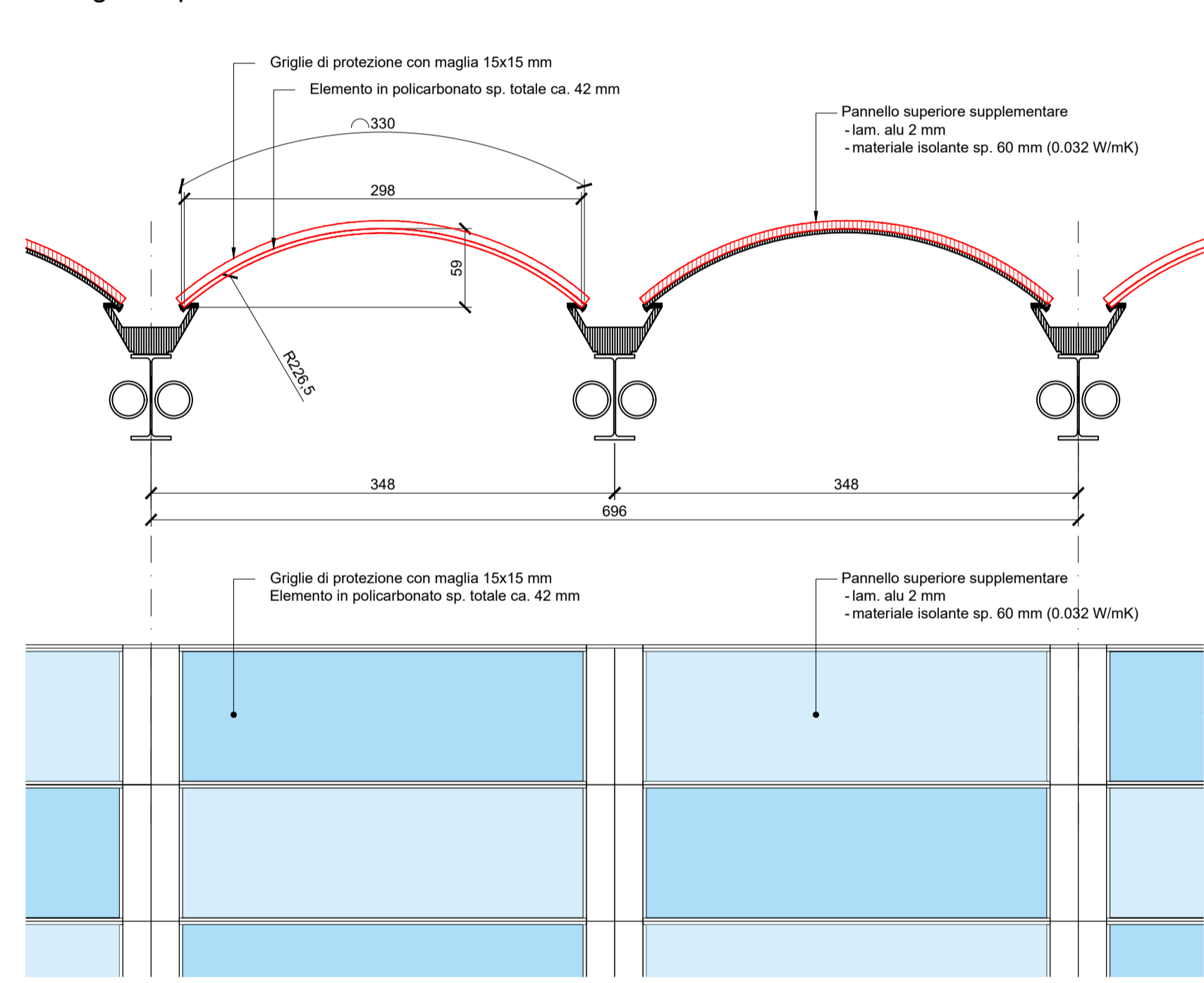
Dettaglio camminamento tra cupole - 1:10
