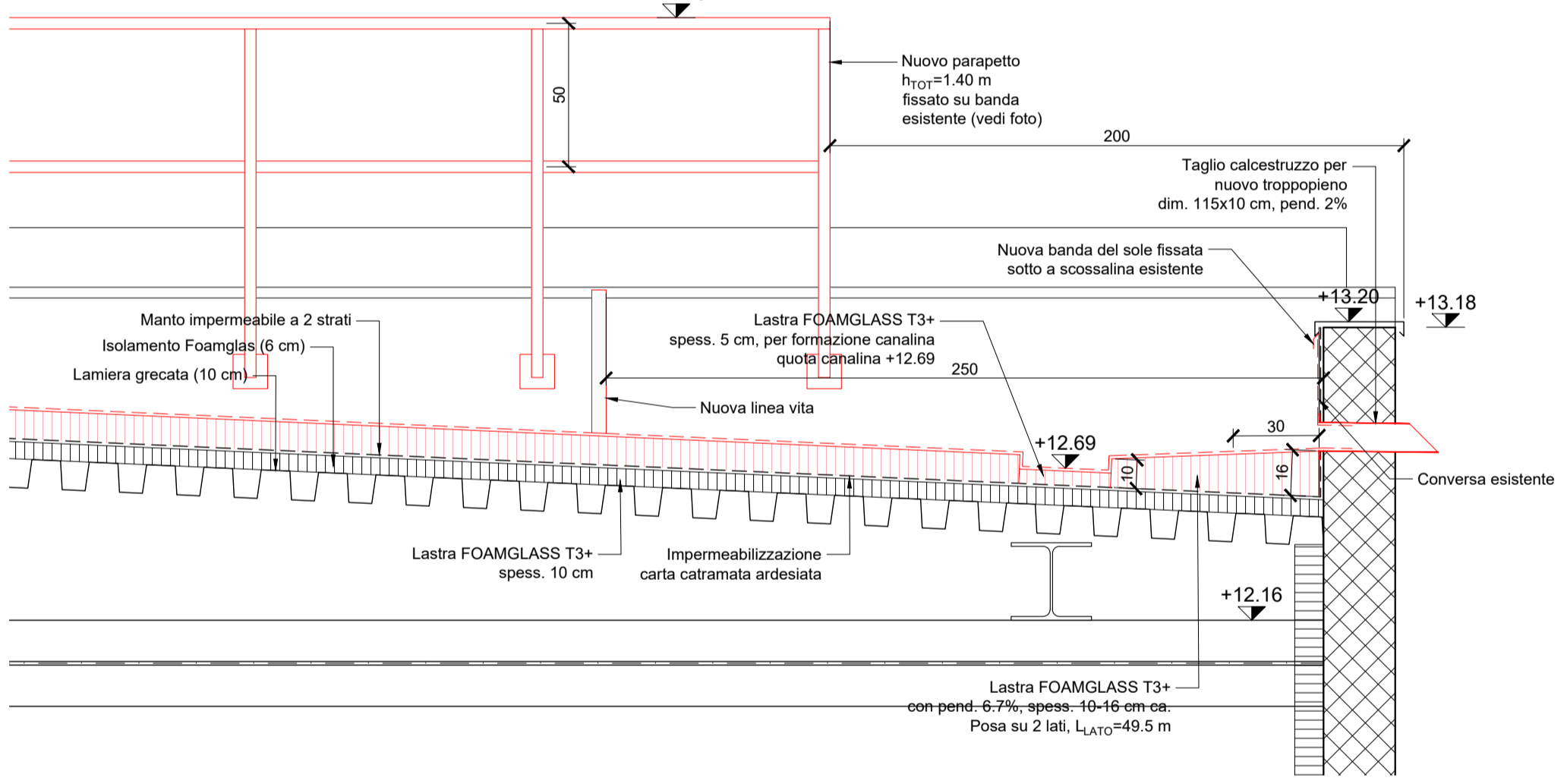
Dettaglio E - Nuovo troppipieno e parapetto - 1:20
