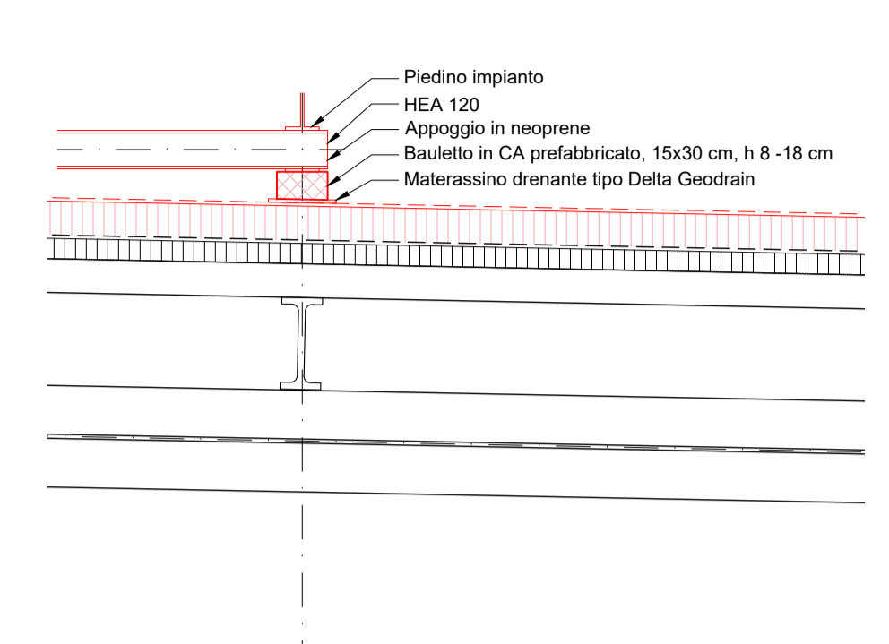
Dettaglio B - Travi d'appoggio impianti - 1:20
