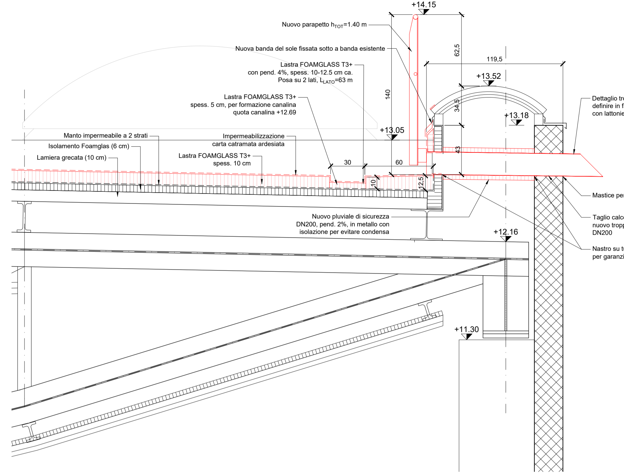
Dettaglio A - Nuovo troppipieno di sicurezza - 1:20
