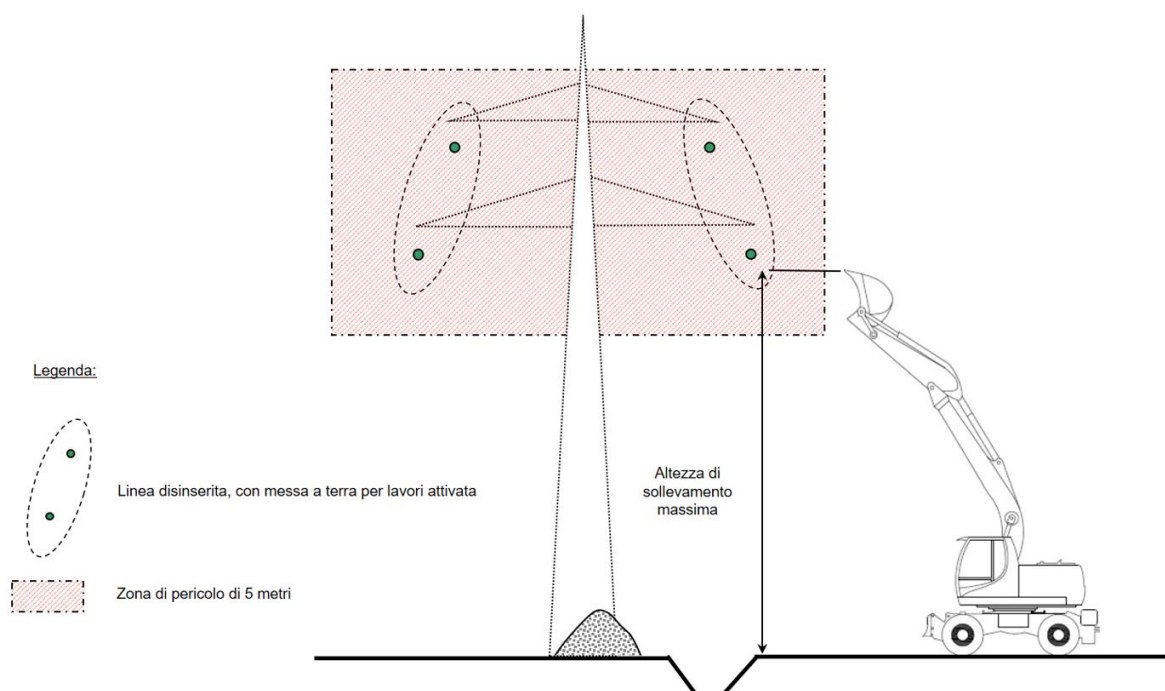
Figura 15: Lavori di costruzione/forestali in prossimità di linee elettriche disinserite e all'interno della zona di pericolo di 5 metri con messa a terra per lavori
