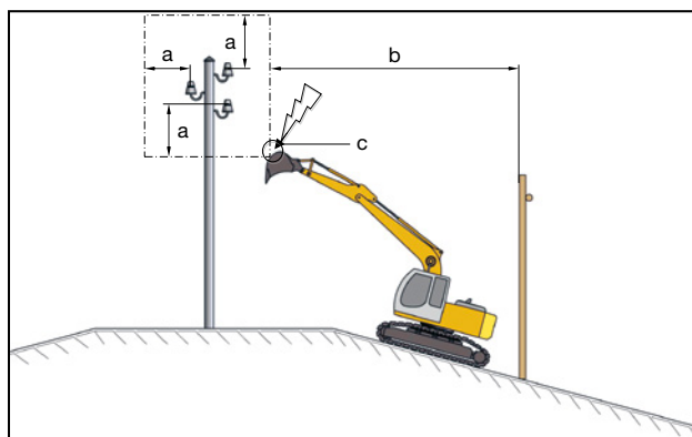
8 a zona vietata a seconda della tensione (vedi figg. 1 – 3) b distanza tra l'asta di protezione e la zona vietata c benna che invade la zona vietata
