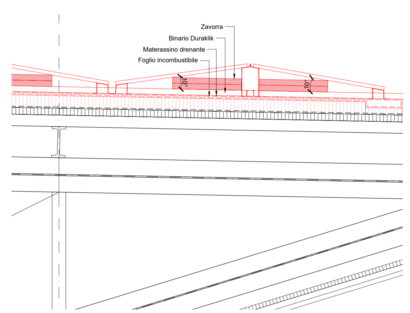
Dettaglio D - Posa impianto fotovoltaico - 1:20
