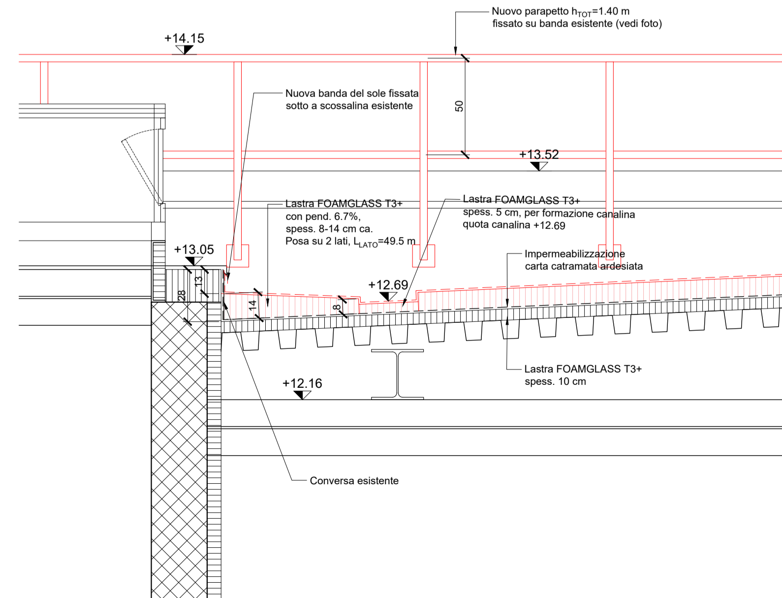
Dettaglio F - Raccordo a tetto piscina - 1:20
