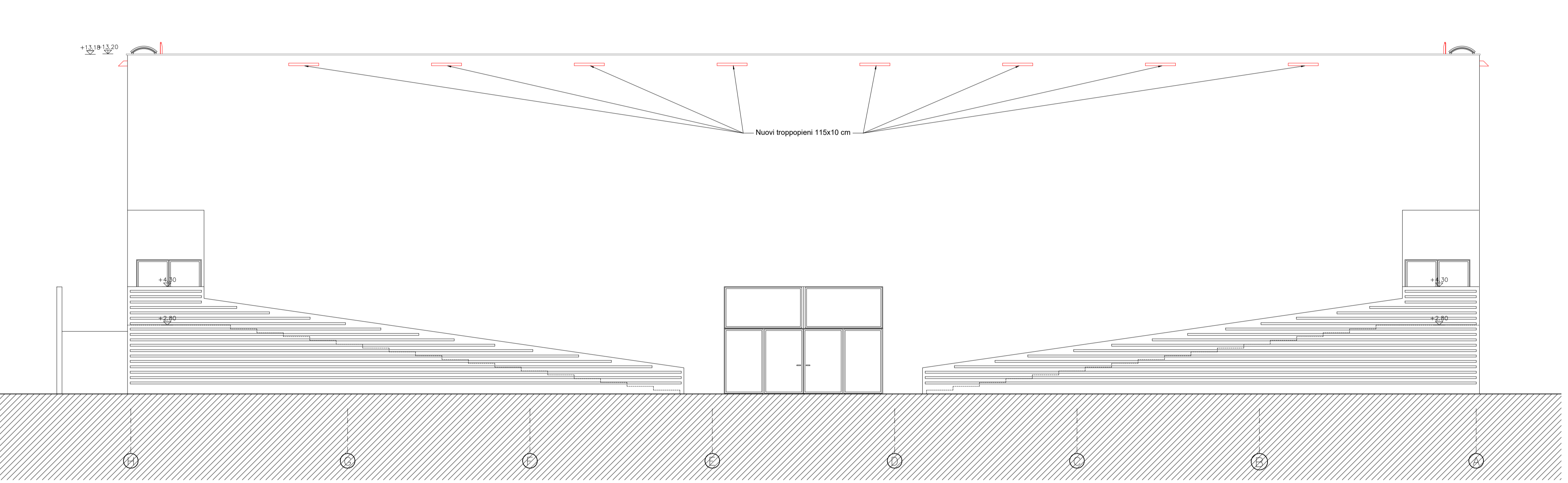
Facciata sud - 1:100
