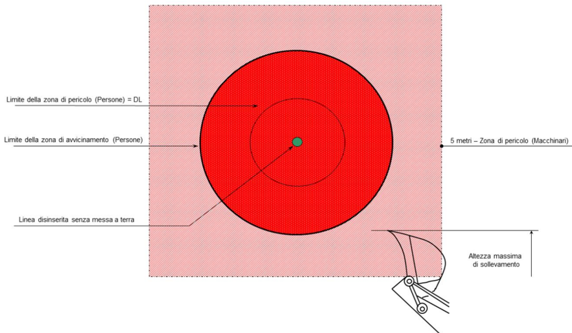
Figura 17: Lavori di costruzione/forestali in prossimità di linee elettriche disinserite e all'interno della zona di pericolo di 5 metri senza messa a terra per lavori e sotto supervisione continua
