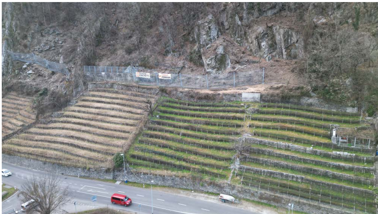
Foto 3: panoramica opere di protezione tra i mappali no. 6343 e 4587
