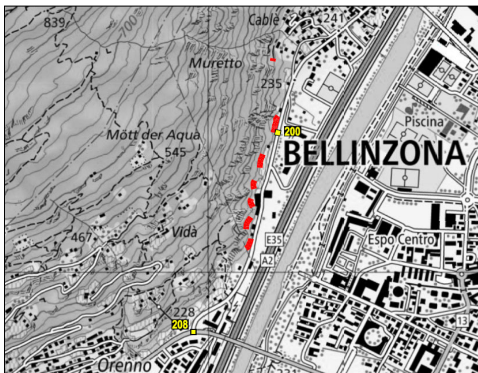
Planimetria orientativa opere di premunizione
