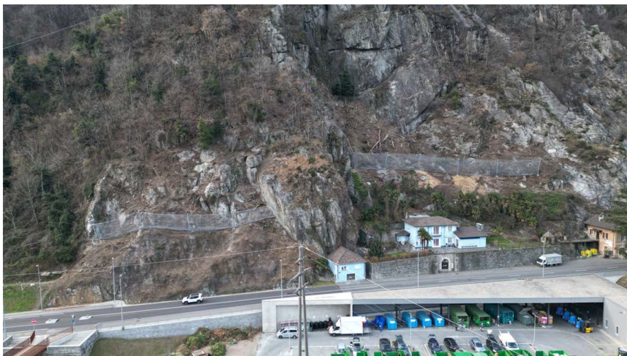
Foto 1: reti paramassi a protezione della strada cantonale e dell'abitazione primaria al mappale no. 3521
