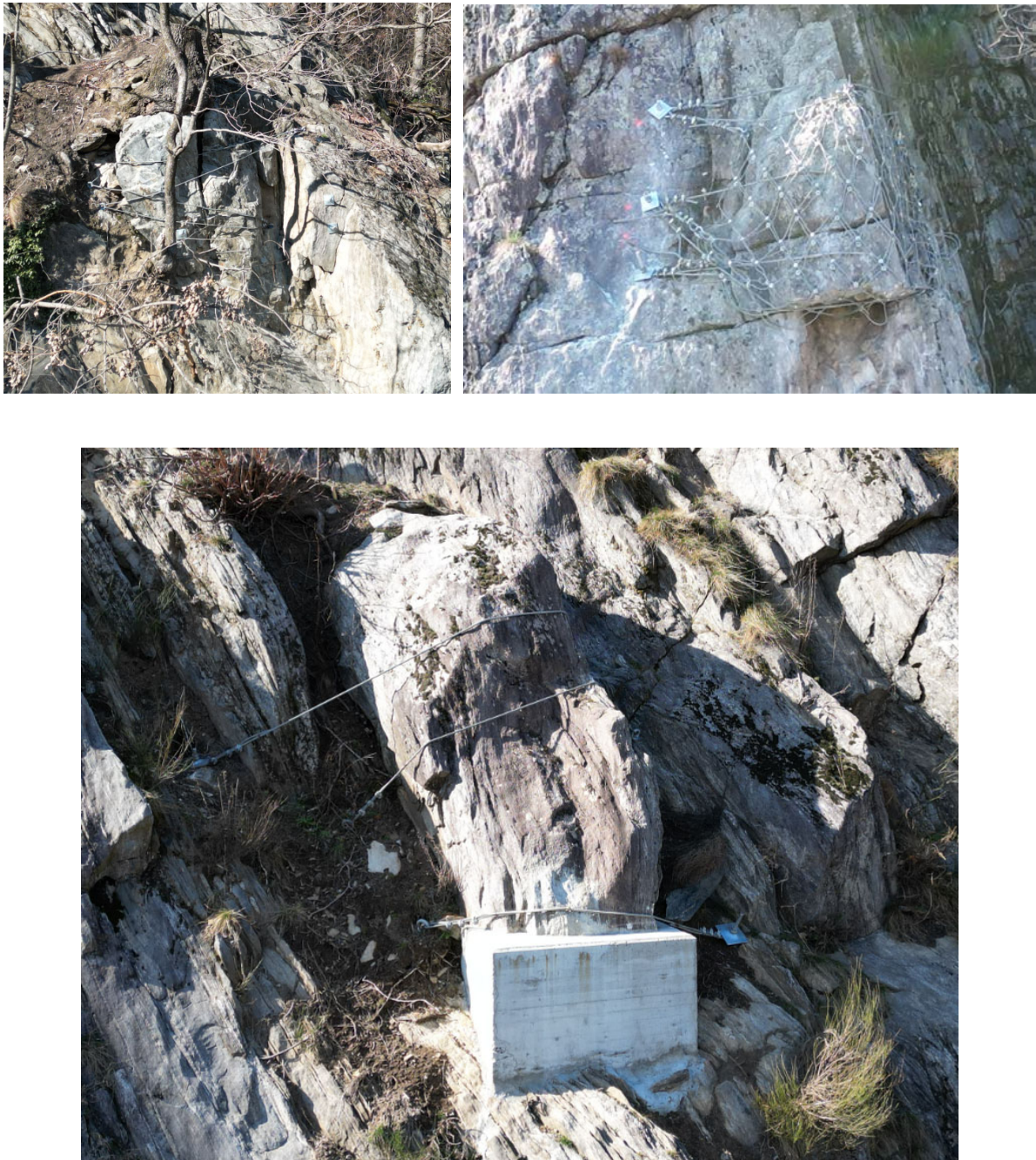
Foto 5: esempi di interventi puntuali di assicurazione attiva in parete
