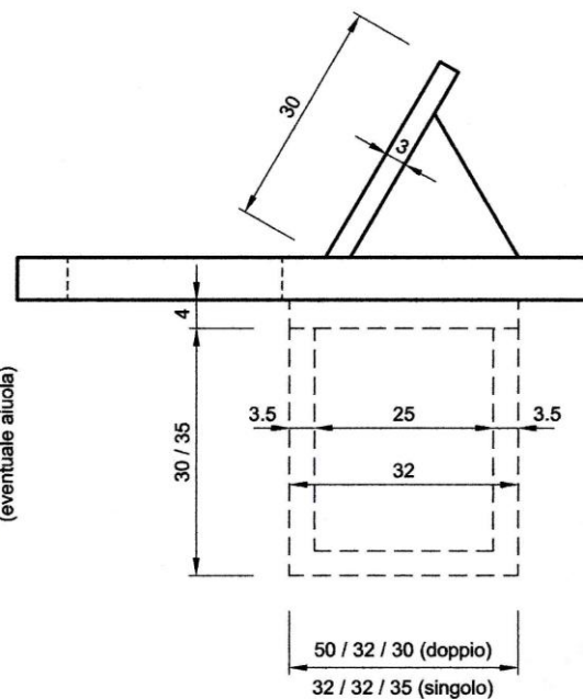
Sezione A - A
